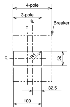
Front-panel cutout
