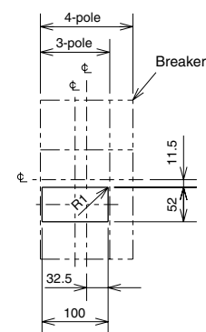
Front-panel cutout
