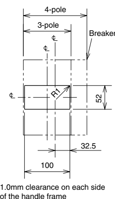
Front-panel cutout
