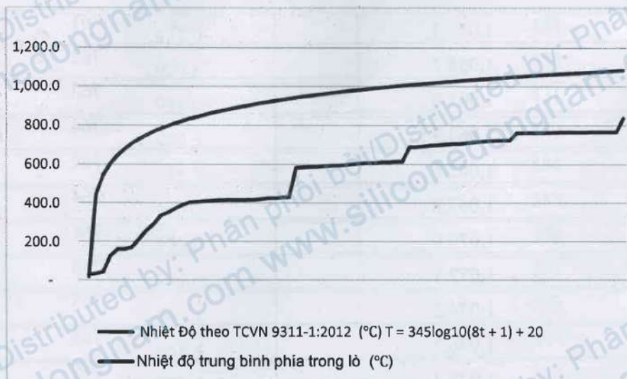
Hình 1. Biểu đồ thể hiện nhiệt độ lò nhiệt trong thời gian đốt so sánh nhiệt độ lý thuyết tính toán
