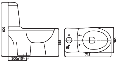
Bàn cầu 2 khối VI107 3.080.000 VNĐ
