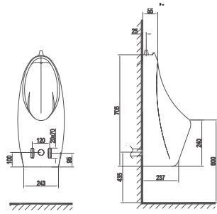
Tiểu nam treo tường T9 ( Cấp dương ) 2.280.000 VNĐ Cấp dương, Nano Titan, gá GT9D, gôm gioăng xả, nút cao su
