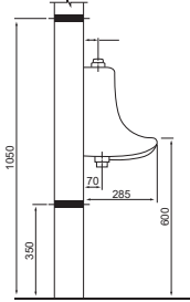
Tiểu nam treo tường TT1 580.000 VNĐ
