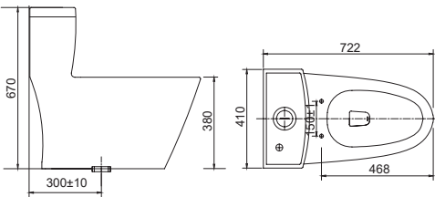
Bàn cầu 1 khối V62 6.160.000 VNĐ
