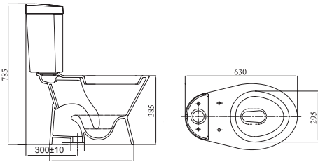
Bàn cầu 2 khối VI66 (Nắp êm V116 + VG826) 3.080.000 VNĐ VI66 (Nắp V1102) 2.780.000 VNĐ
