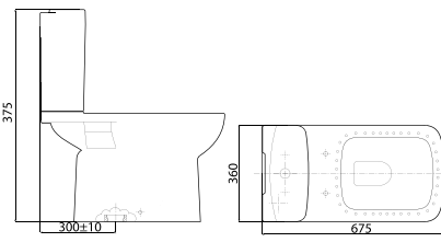
Bàn cầu 2 khối VI6 3.550.000 VNĐ
