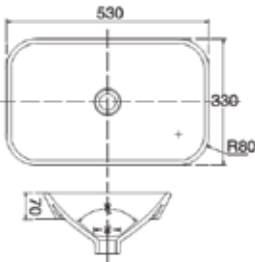
Chậu đặt bàn V28 1.290.000 VNĐ
