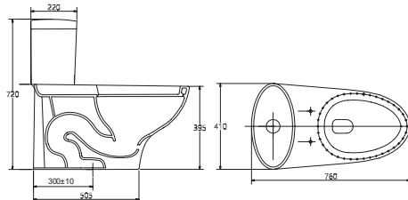
Bàn cầu 1 khối V37M 4.250.000 VNĐ V37S 4.250.000 VNĐ
