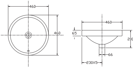
Chậu bán dương bàn CD6 1.080.000 VNĐ
