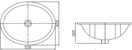
Chậu âm bàn CA2 1.500.000 VNĐ
