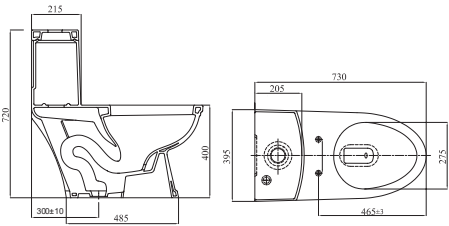
Bàn cầu 1 khối V39 4.080.000 VNĐ V39M 4.300.000 VNĐ
