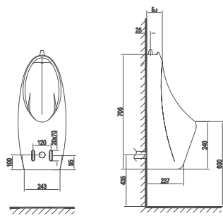
Tiểu nam treo tường T9 ( Cấp âm ) 2.660.000 VNĐ Cấp âm, Nano Titan, gá GT9A, cụm gioăng xả, nút cao su
