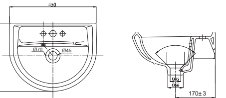
Chậu treo tường VTL3N 580.000 VNĐ
