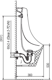
Tiểu nam treo tường T6 ( Cấp âm ) 3.260.000 VNĐ Cấp âm, Nano Titan, gá , cụm gioăng xả, nút cao su
