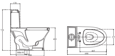
Bàn cầu 1 khối V45M 4.880.000 VNĐ
