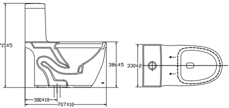
Bàn cầu 1 khối V35M 5.350.000 VNĐ
