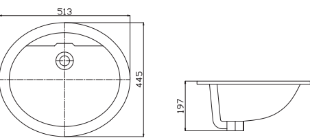
Chậu dương vành CD1 1.080.000 VNĐ
