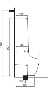
Tiểu nam đặt sàn BS604 7.260.000 VNĐ
