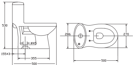
Bàn cầu 1 khối (Trẻ em) BTE 2.450.000 VNĐ
