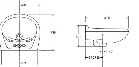
Chậu treo tường VTL3 580.000 VNĐ
