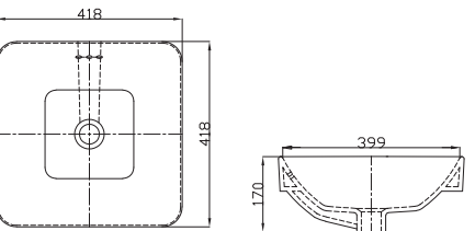
Chậu bán dương bàn CD20 1.320.000 VNĐ
