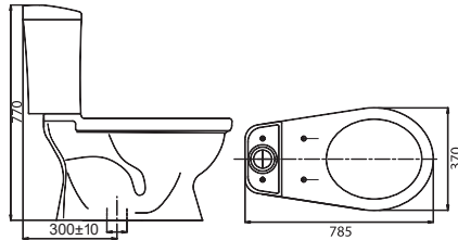
Bàn cầu 2 khối, xả 1 nhấn VI28 2.600.000 VNĐ
