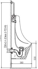
Tiểu nam treo tường T6 ( Cấp dương ) 3.080.000 VNĐ Cấp dương, Nano Titan, gá , cụm gioăng xả, nút cao su
