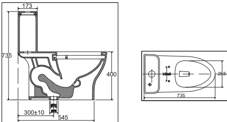
Bàn cầu 1 khối V63 5.990.000 VNĐ
