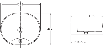
Chậu đặt bàn CD19 1.700.000 VNĐ
