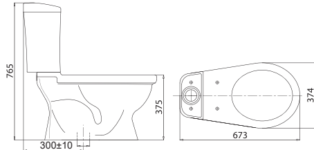
Bàn cầu 2 khối VI88 (Nắp êm V116 + VG826) 3.080.000 VNĐ VI88 (Nắp V1102) 2.780.000 VNĐ
