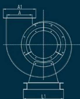
Kích thước cửa hút
