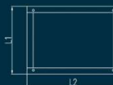
Kích thước cửa thổi
